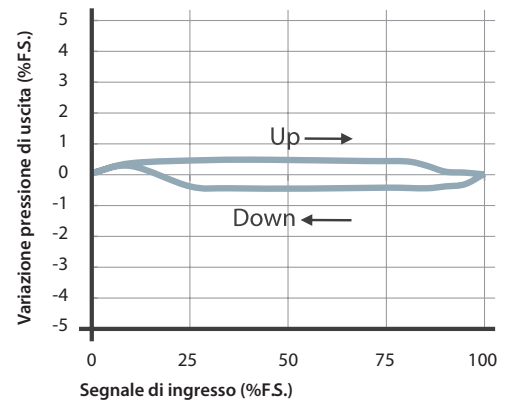
Caratteristica pressione
