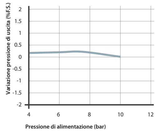
Caratteristica pressione
