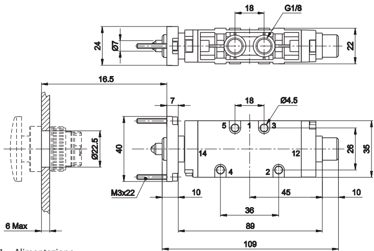
5/2 G1/8
