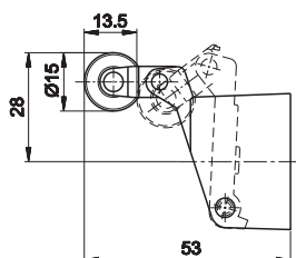
C LEVA RULLO LATERALE BIDIREZIONALE G1/8
