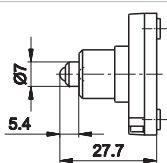
E PUNTALE A RULLO CON PROTEZIONE ANTIPOLVERE G1/8
