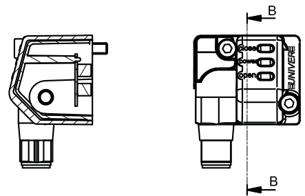
B-B ( 1 : 1 )
